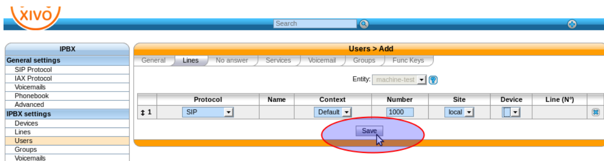
Fig. 1.13: Save
