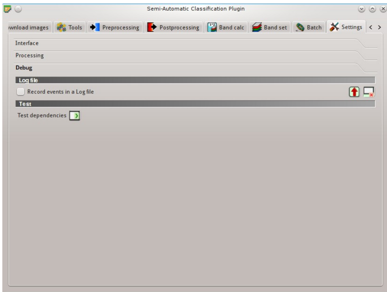
Rys. 10.40: Debug
