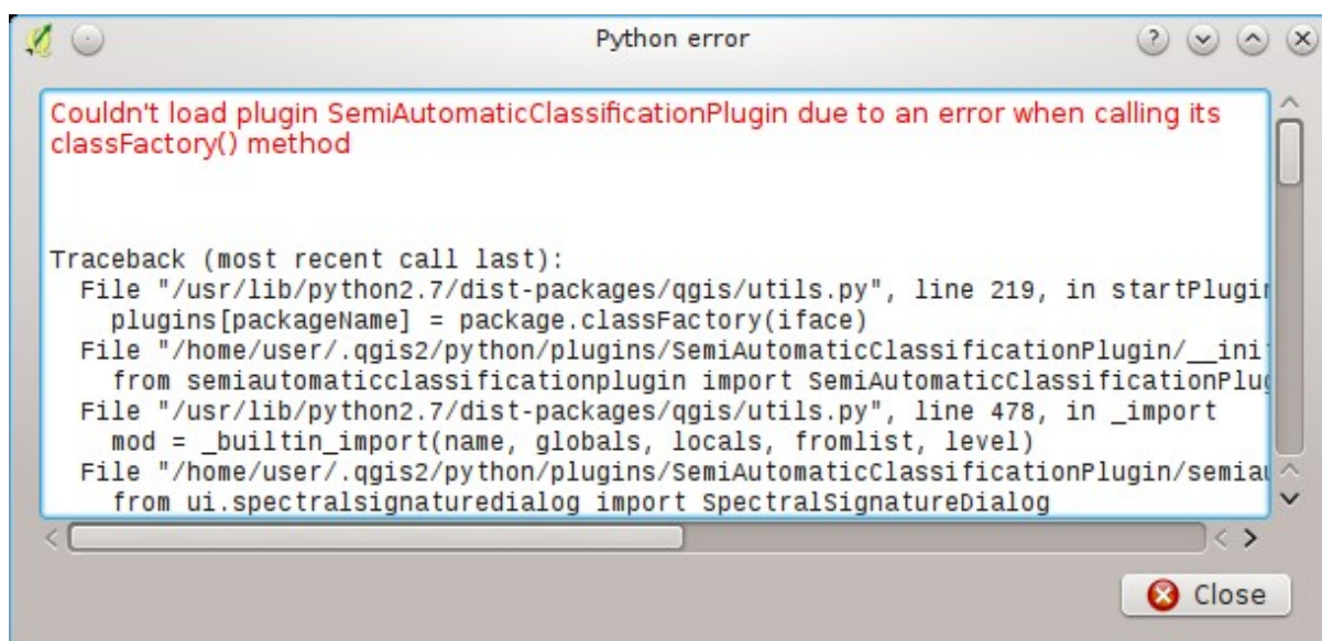
Rys. 29.2: Error message
