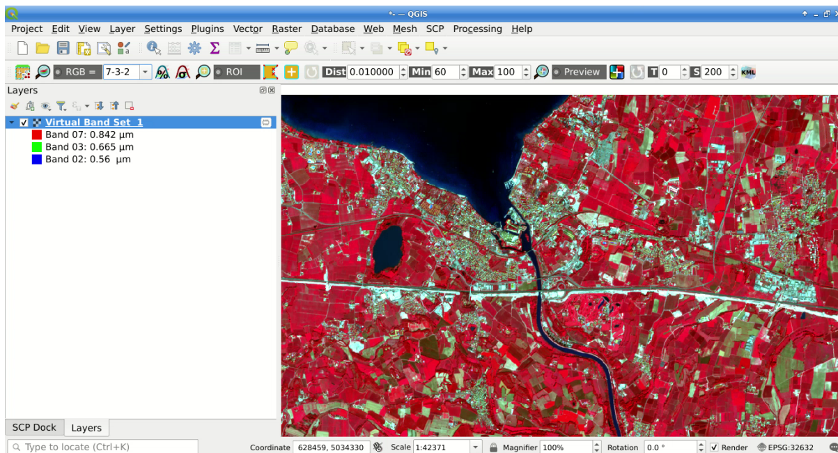
Рис. 2: Color composite RGB=7-3-2
