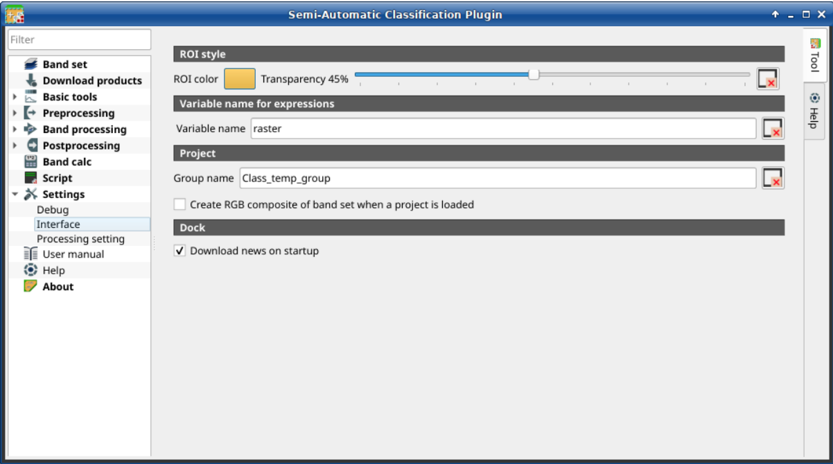
Rys. 48: Interface
