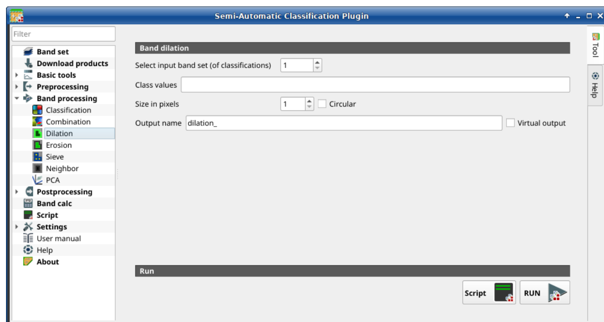
Rys. 35: Dilation
