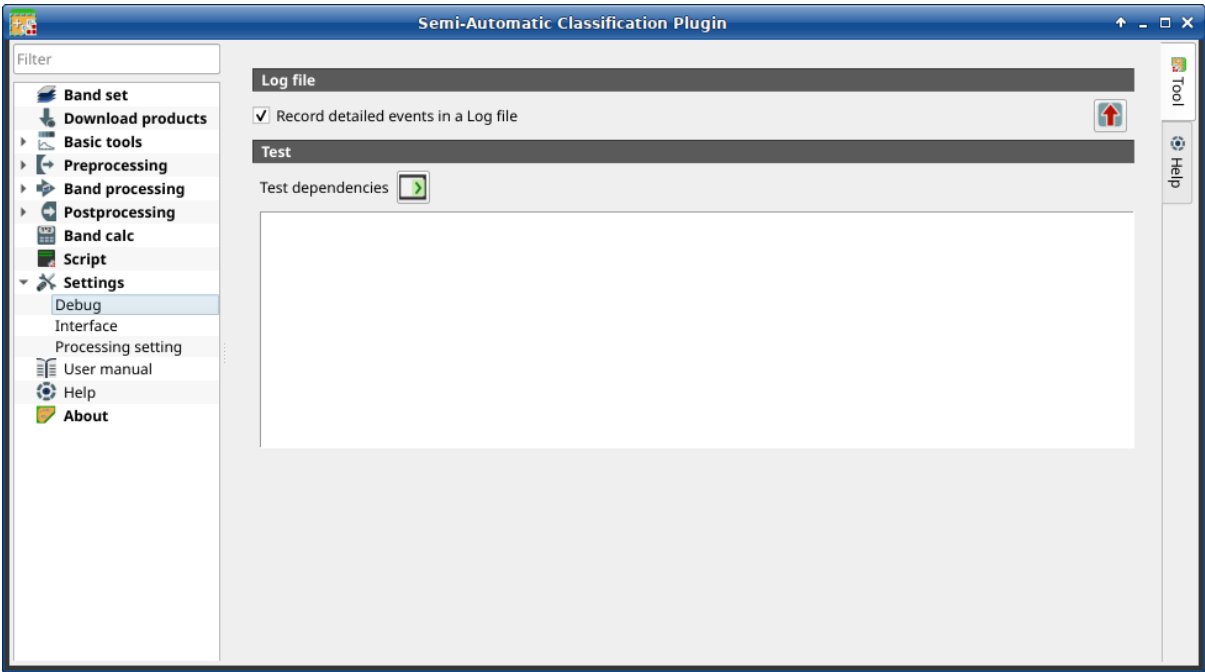
Rys. 47: Debug
