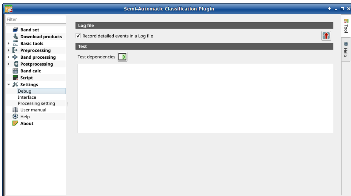
Rys. 1: Debug
