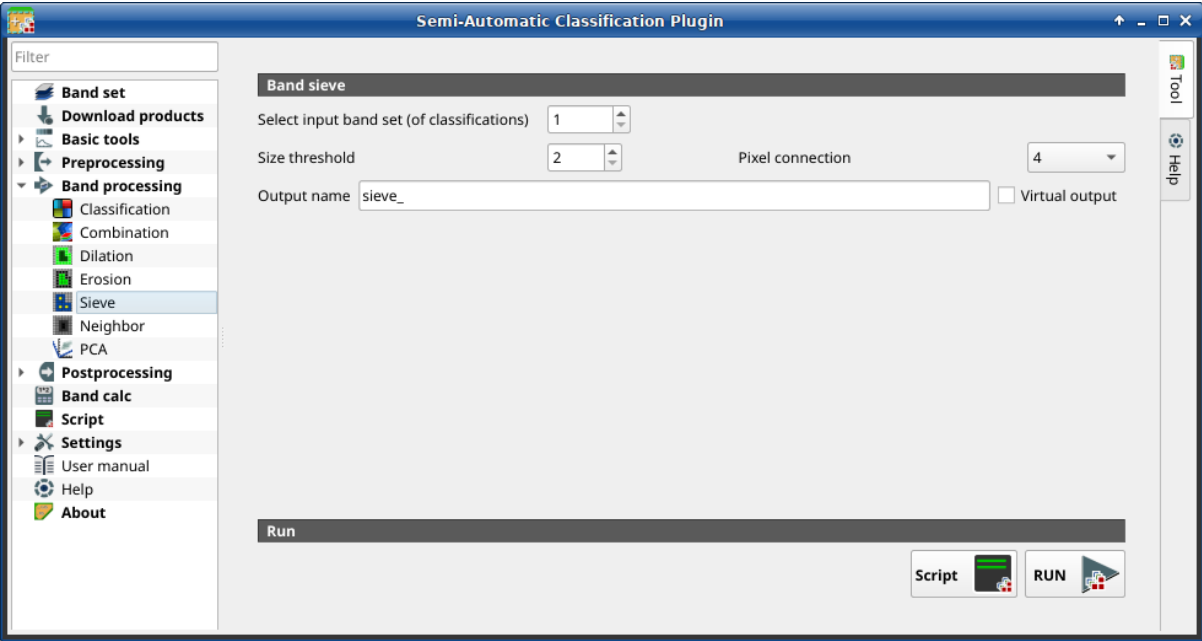
Rys. 37: Sieve
