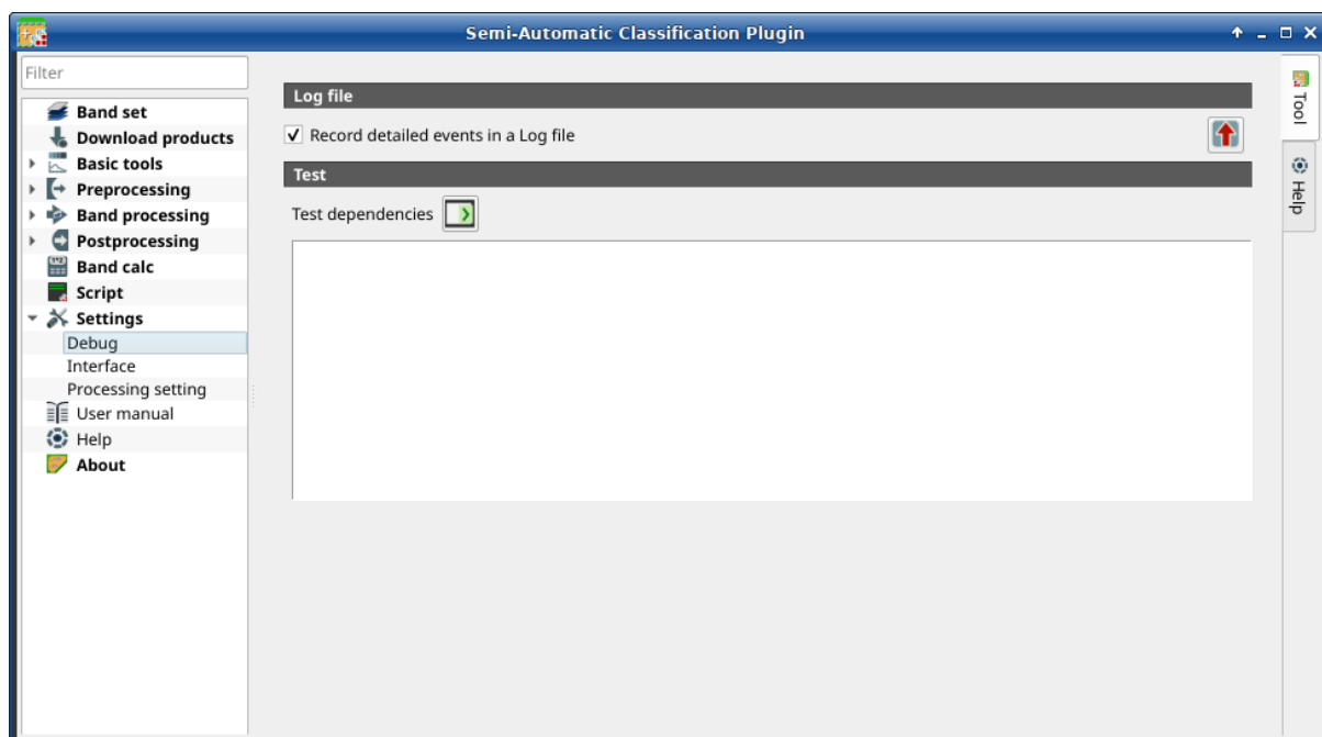
1: Debug
