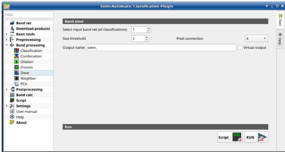
37: Sieve
