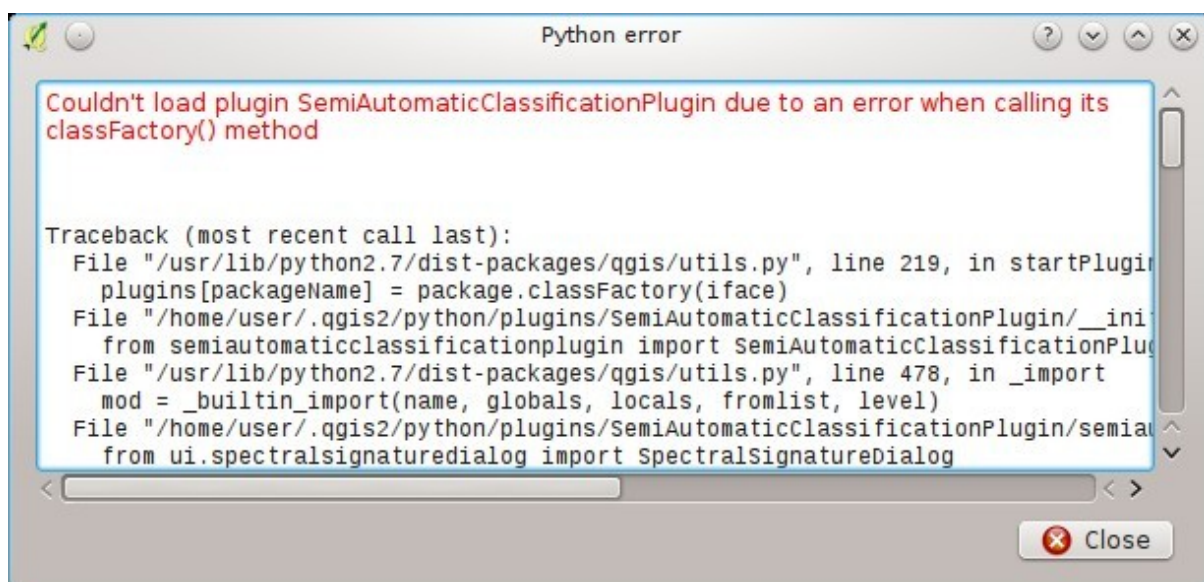
2: Error message
