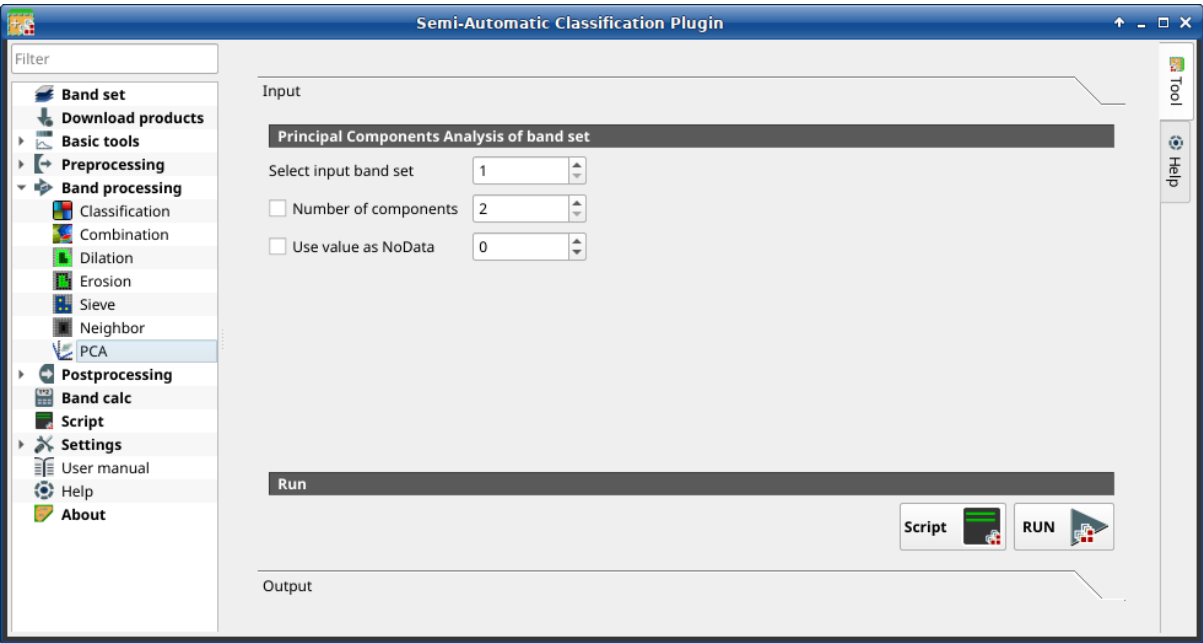
39: PCA
