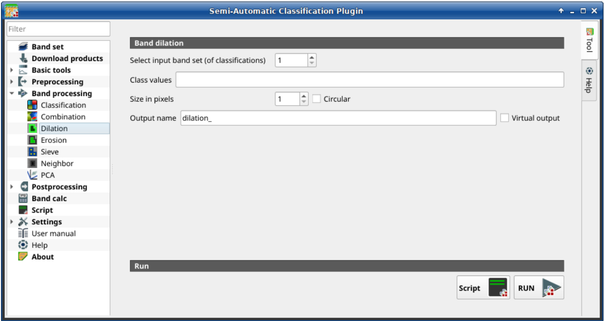
35: Dilation
