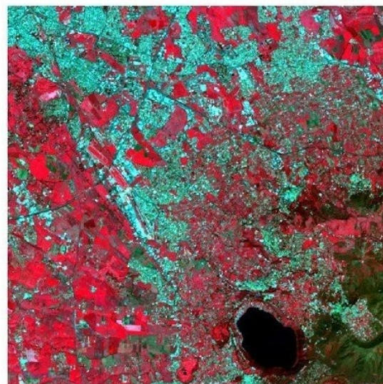
RGB = 543
