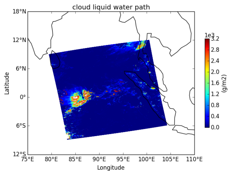
Fig. 10: Cloud CCI
