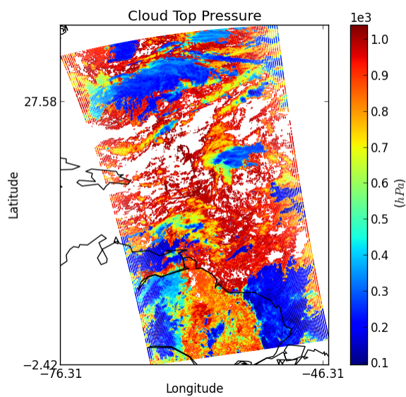
Fig. 3: MODIS Level 2
