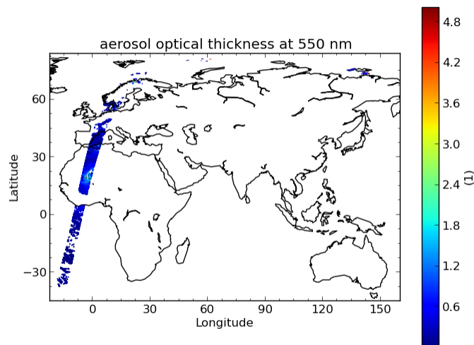
Fig. 9: Aerosol CCI
