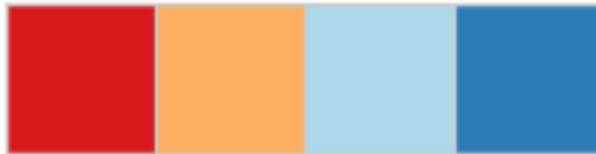
RdYIBu - 4
