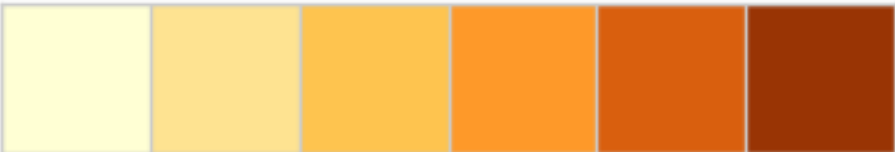
YIOrBr - 6
